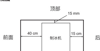
侧视图
