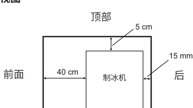
侧视图
