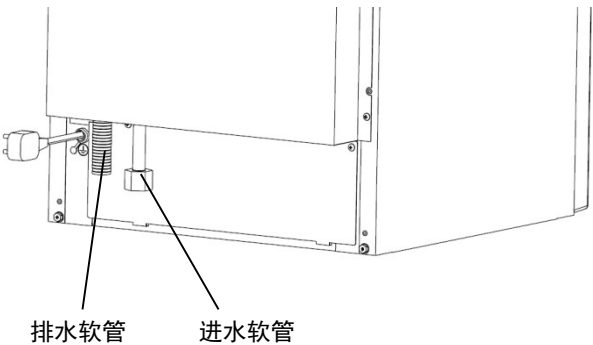
[SRM-100B]
